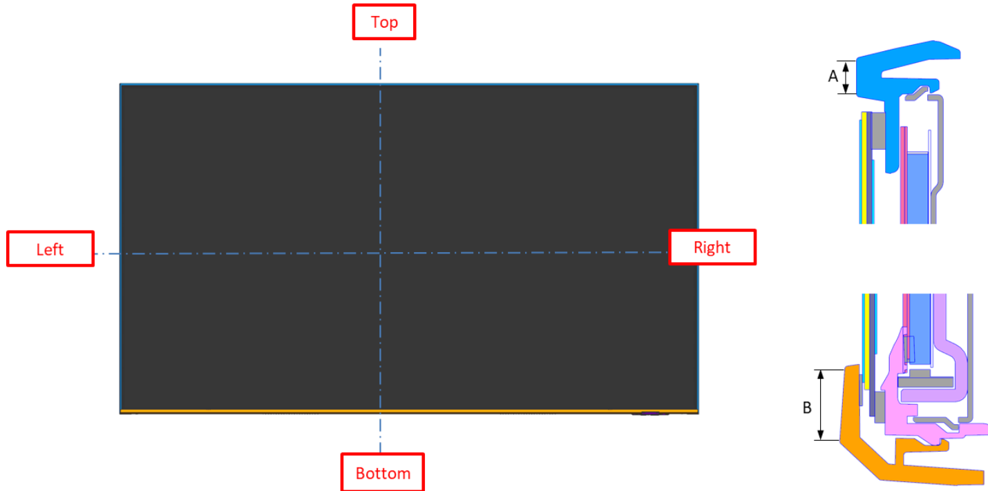
Q60C Bezel Dimensions
